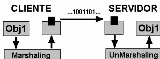
Figura A.6: Serialização de Objetos
