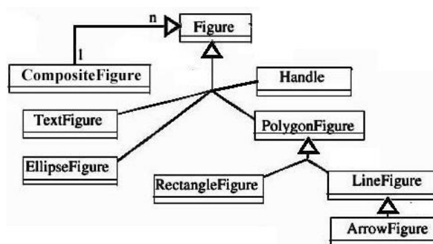
Figura 4.3: Classe Figure e suas subclasses.
