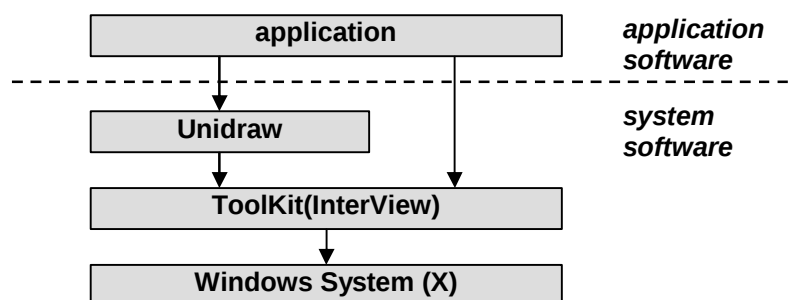
Figura 4.9: Camadas de uma aplicação sob Unidraw [Vlissides,90]..
