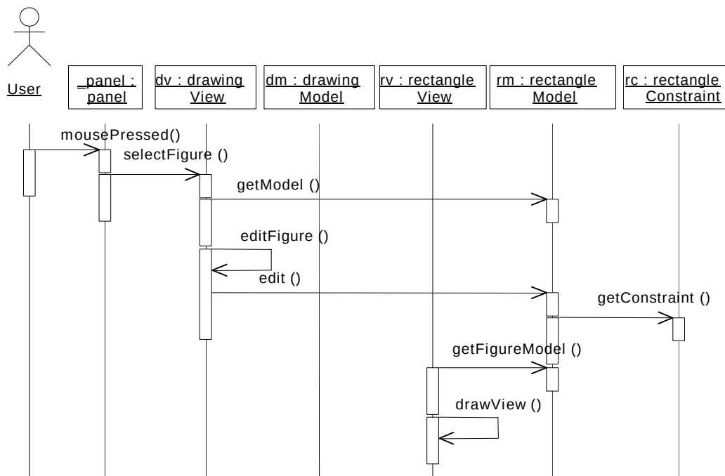
Figura 5.11: Diagrama de Sequência editar figura.
