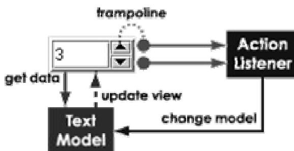
Figura A.3: Modelo de delegação de Eventos[Eckel,00]
