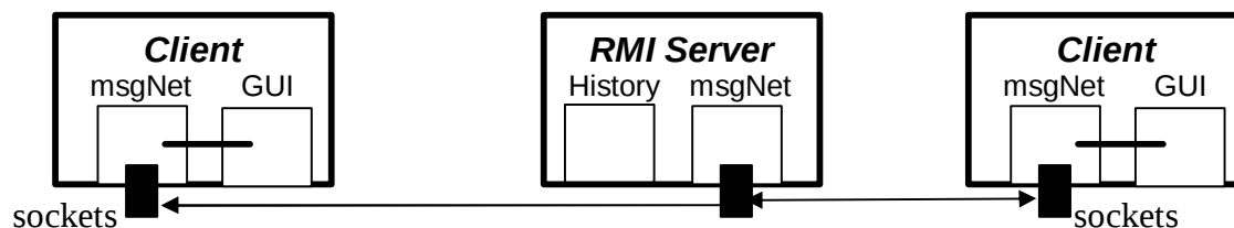
Figura A.5: Abordagem RMI para compartilhamento de objetos.
